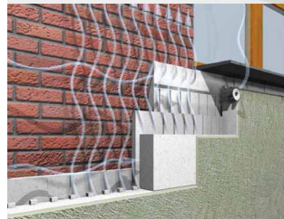
Izodom ventileret panel.
